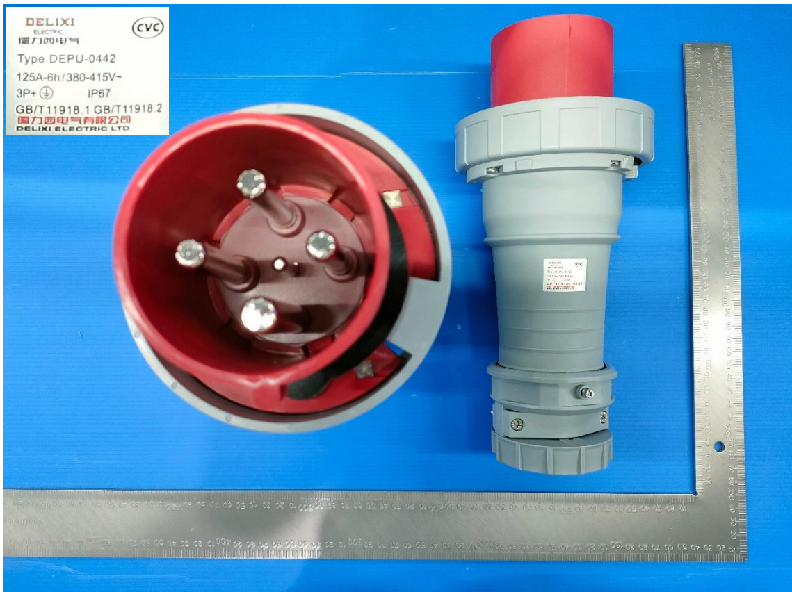
DEPU-0442 125A-6h/415V ~ 3P+PE IP67
