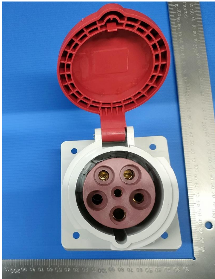
DEPU-435 63A-6h/415V ~ 3P+N+PE IP44
