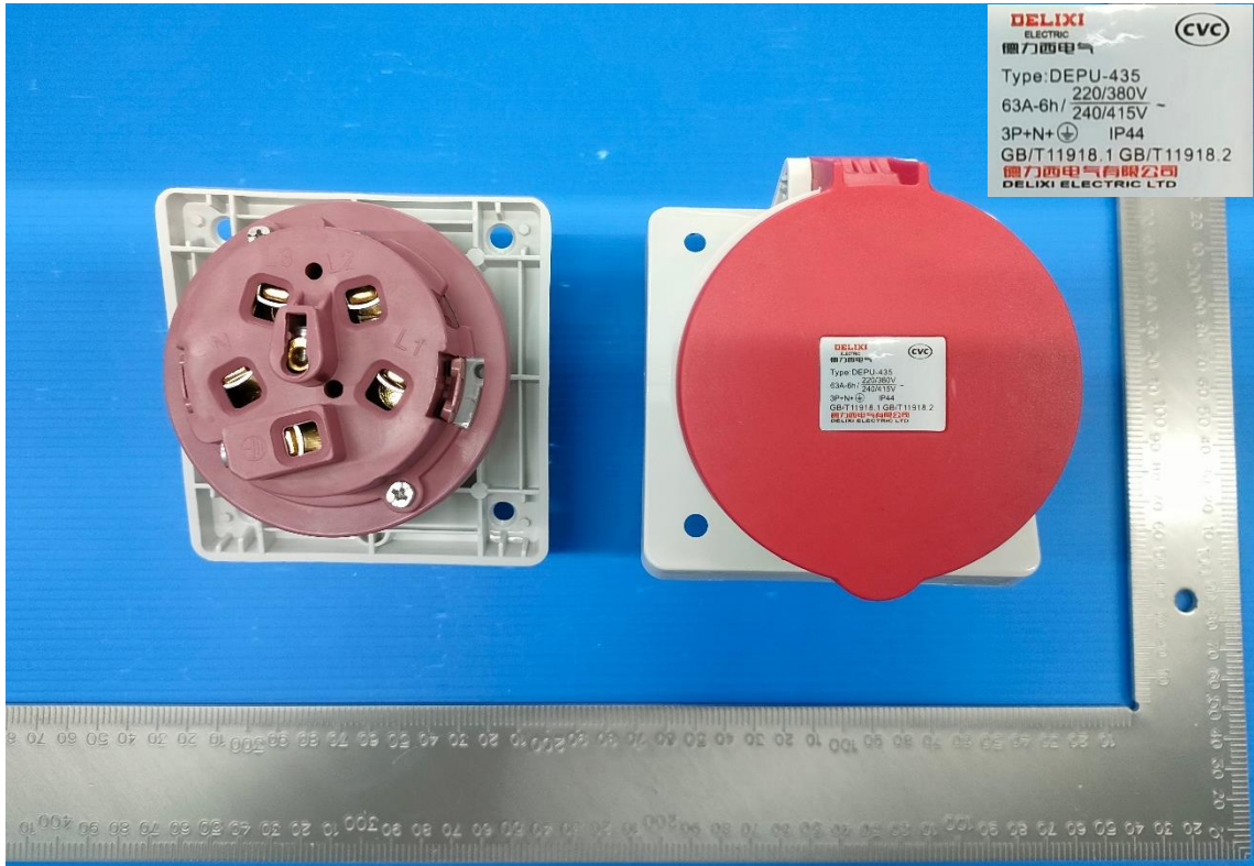
DEPU-435 63A-6h/415V ~ 3P+N+PE IP44
