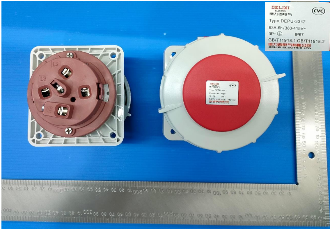
DEPU-3342 63A-6h/415V ~ 3P+PE IP67
