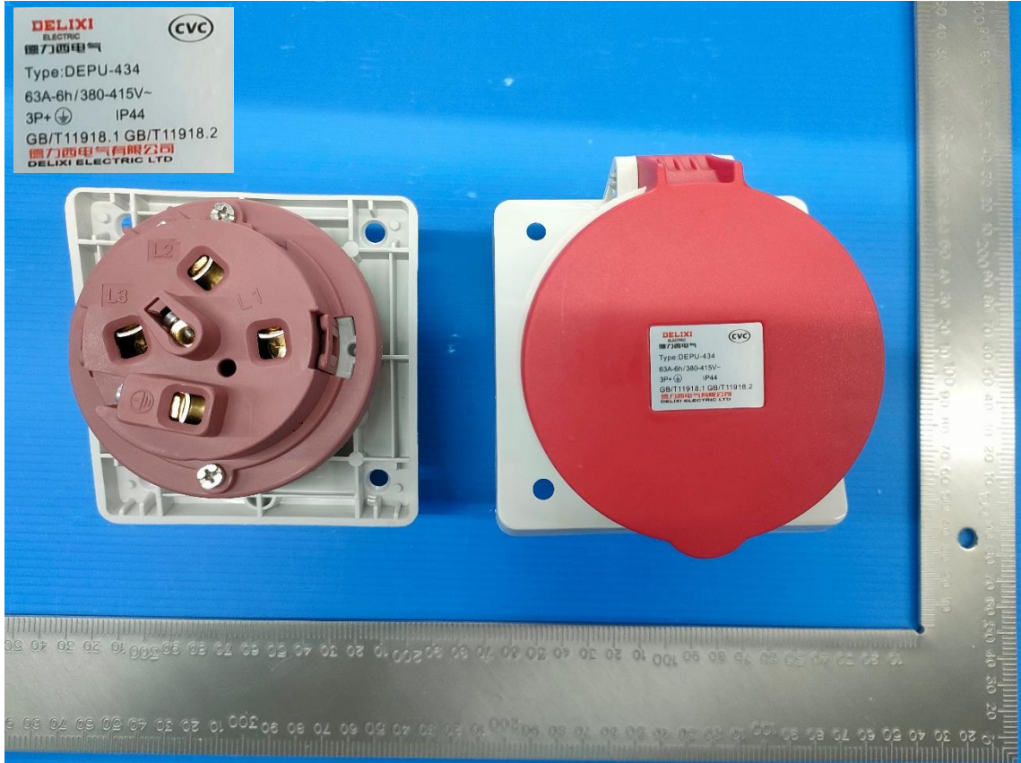
DEPU-434 63A-6h/415V ~ 3P+PE IP44
