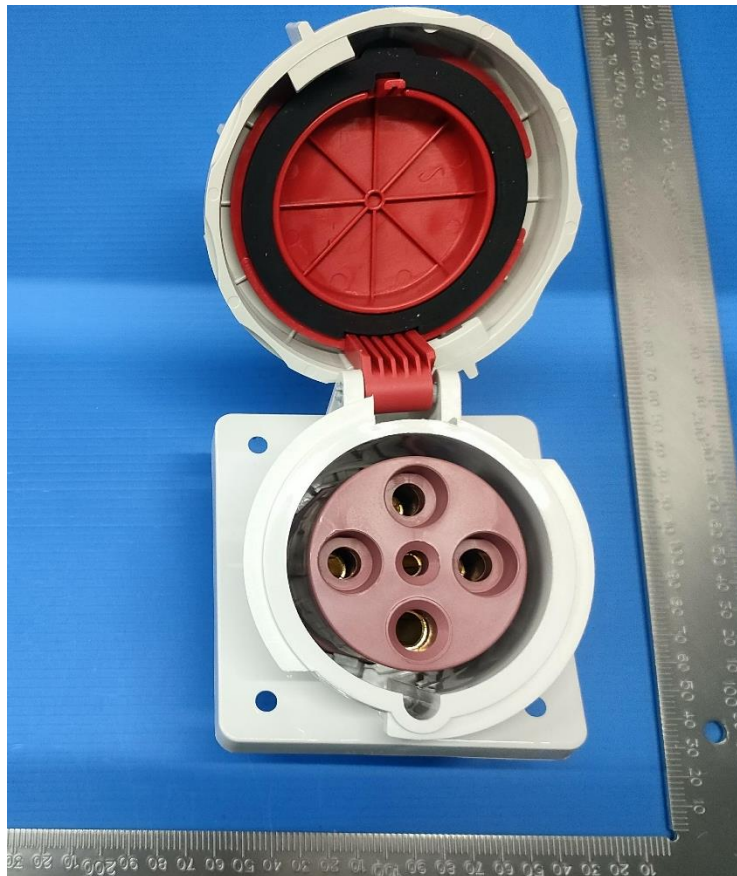
DEPU-4342 63A-6h/415V ~ 3P+PE IP67
