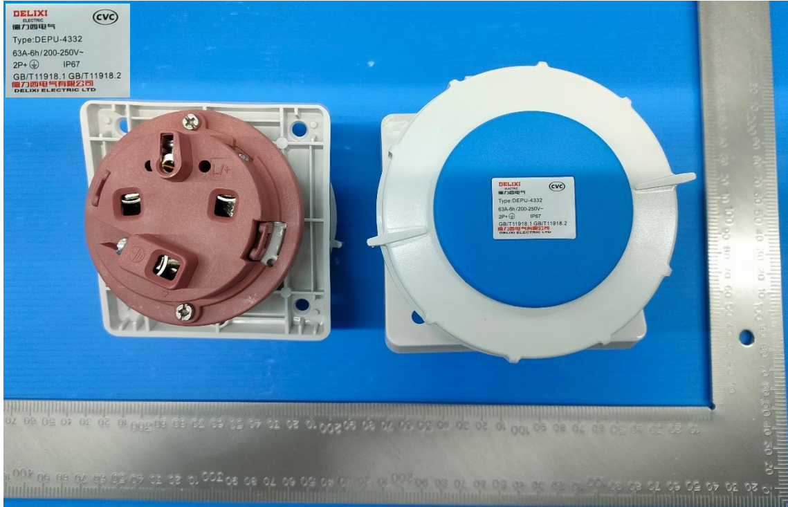
DEPU-4332 63A-6h/250V ~ 2P+PE IP67
