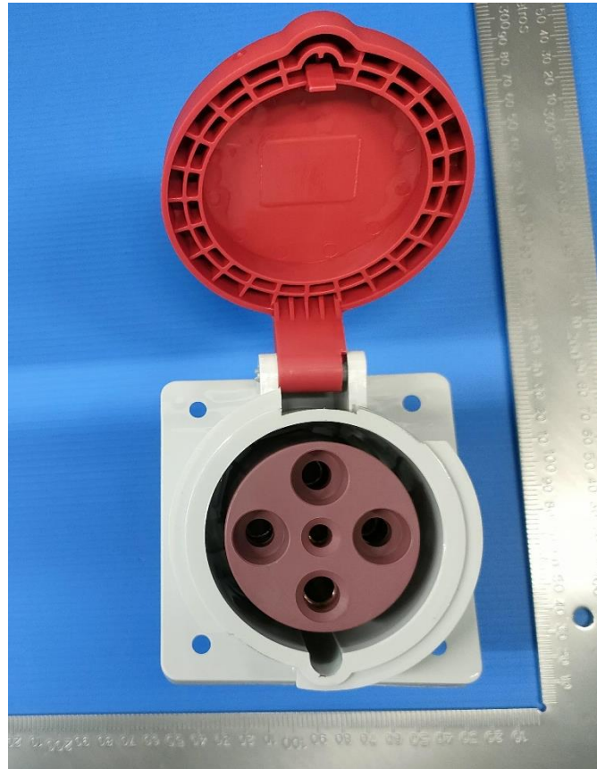
DEPU-434 63A-6h/415V ~ 3P+PE IP44
