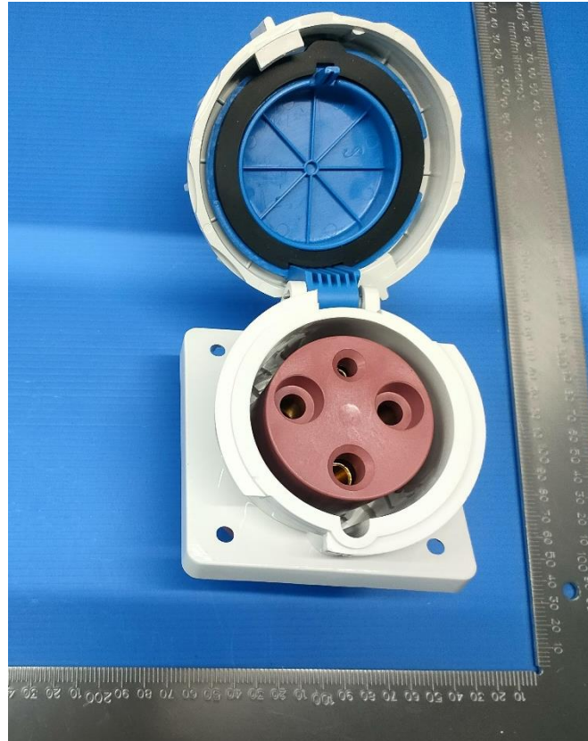
DEPU-4332 63A-6h/250V ~ 2P+PE IP67
