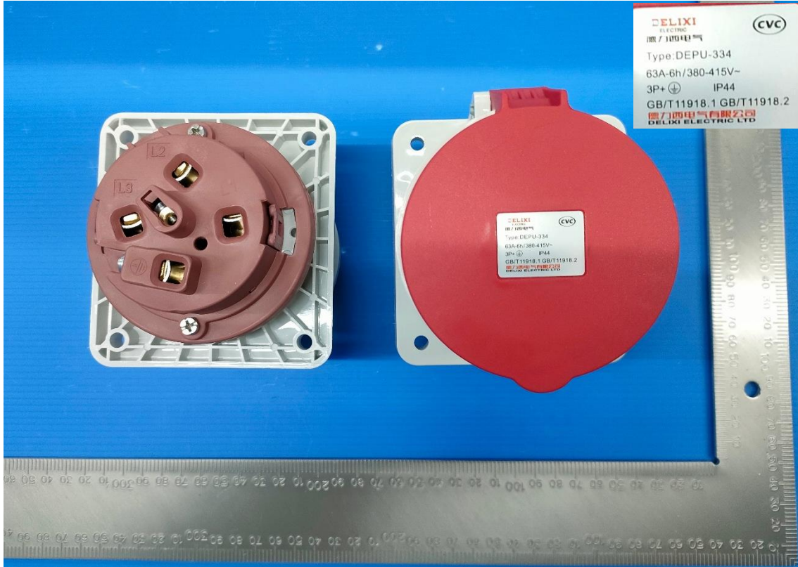
DEPU-334 63A-6h/415V ~ 3P+PE IP44
