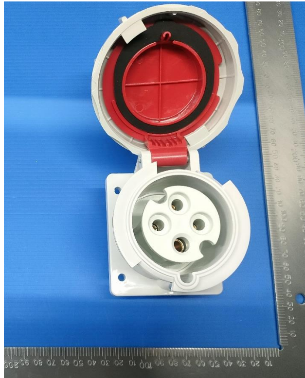
DEPU-3242 32A-6h/415V ~ 3P+PE IP67
