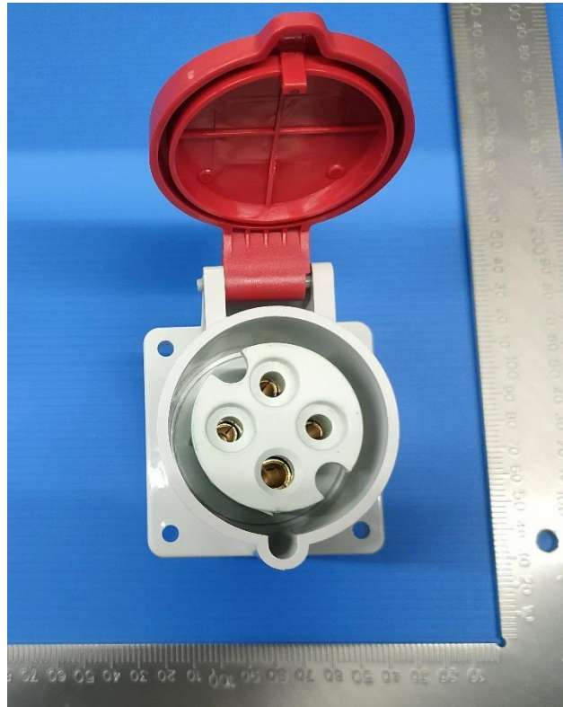
DEPU-324 32A-6h/415V ~ 3P+PE IP44
