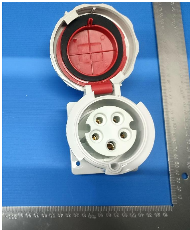
DEPU-3252 32A-6h/415V ~ 3P+N+PE IP67
