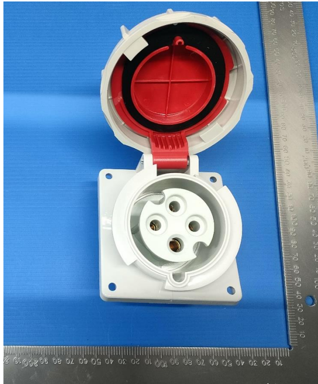
DEPU-4242 32A-6h/415V ~ 3P+PE IP67
