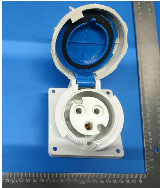
DEPU-4232 32A-6h/250 ~ 2P+PE IP67
