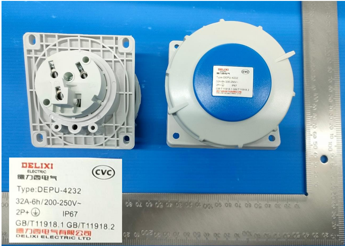
DEPU-4232 32A-6h/250 ~ 2P+PE IP67
