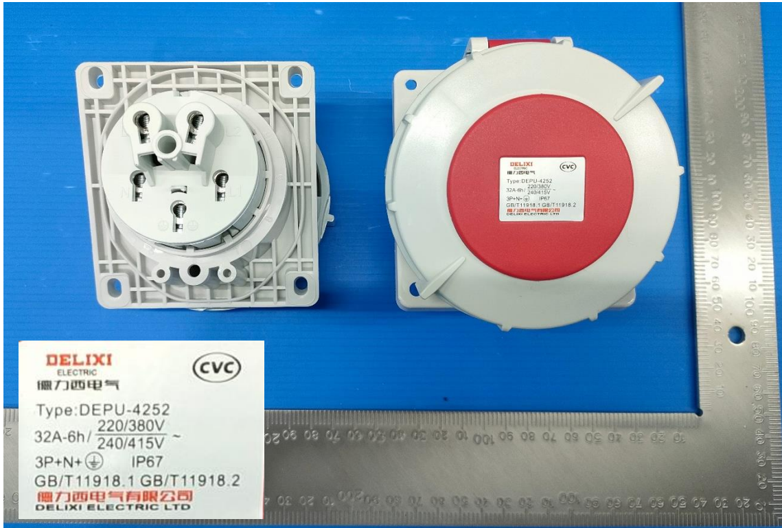
DEPU-4252 32A-6h/415V ~ 3P+N+PE IP67
