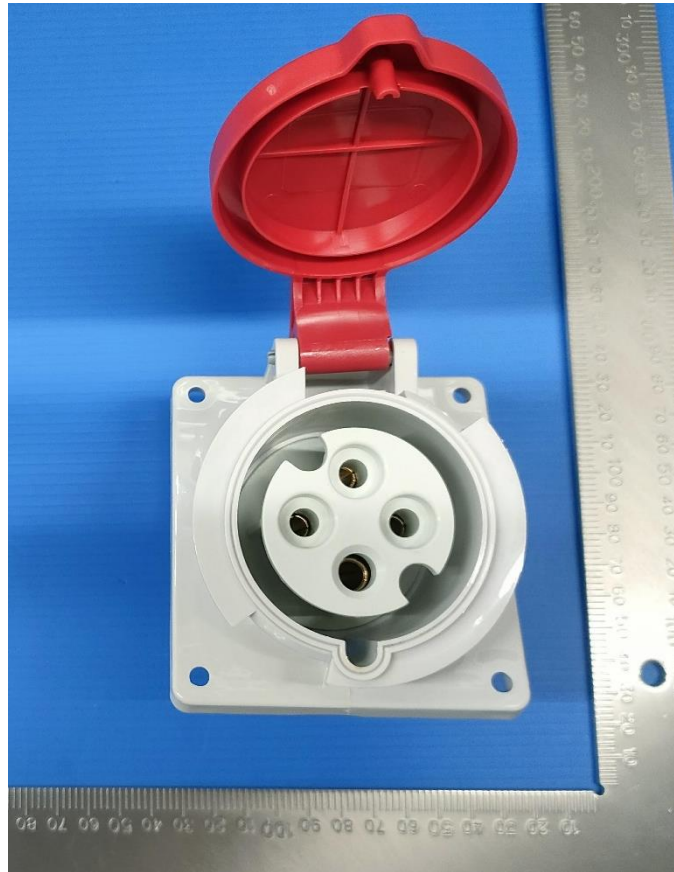
DEPU-424 32A-6h/415V ~ 3P+PE IP44
