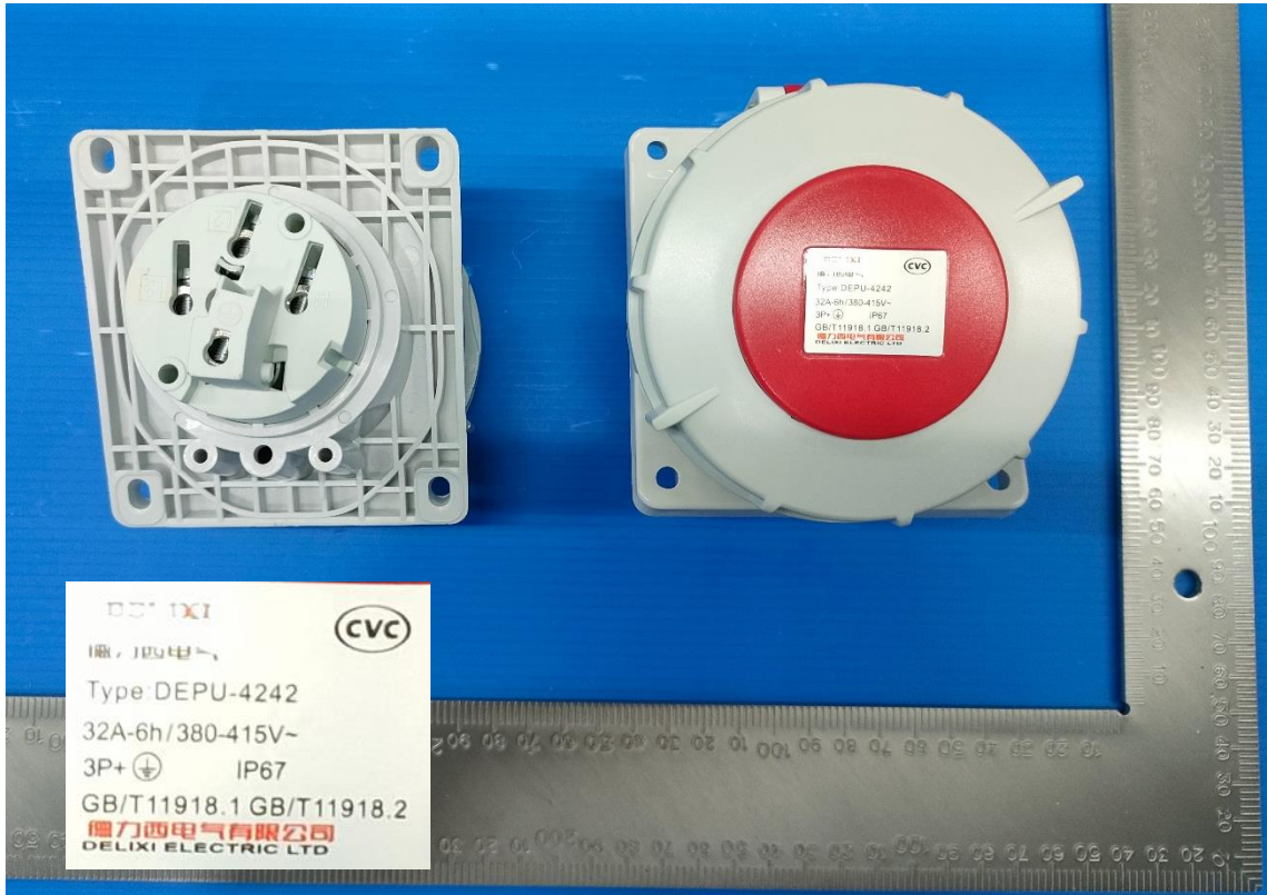
DEPU-4242 32A-6h/415V ~ 3P+PE IP67
