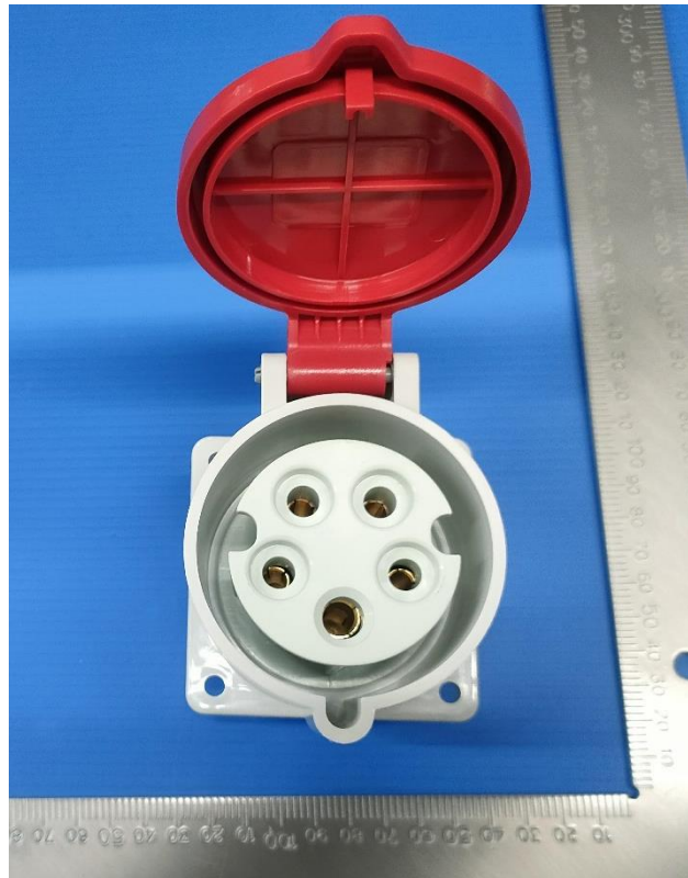
DEPU-325 32A-6h/415V ~ 3P+N+PE IP44
