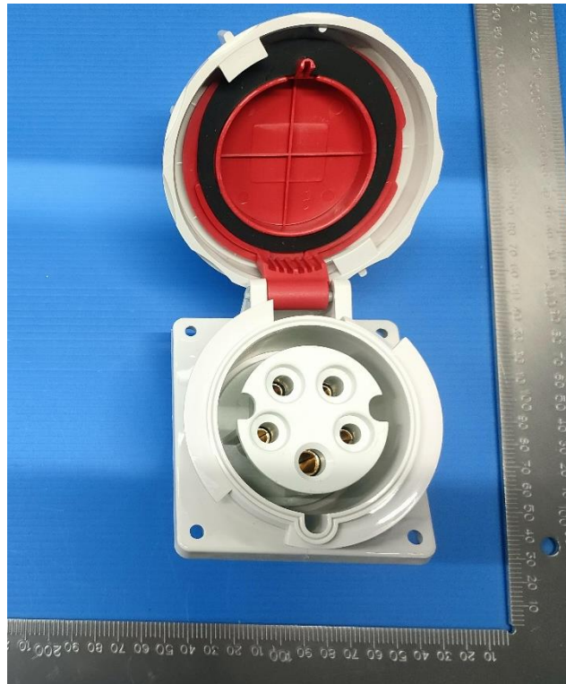
DEPU-4252 32A-6h/415V ~ 3P+N+PE IP67
