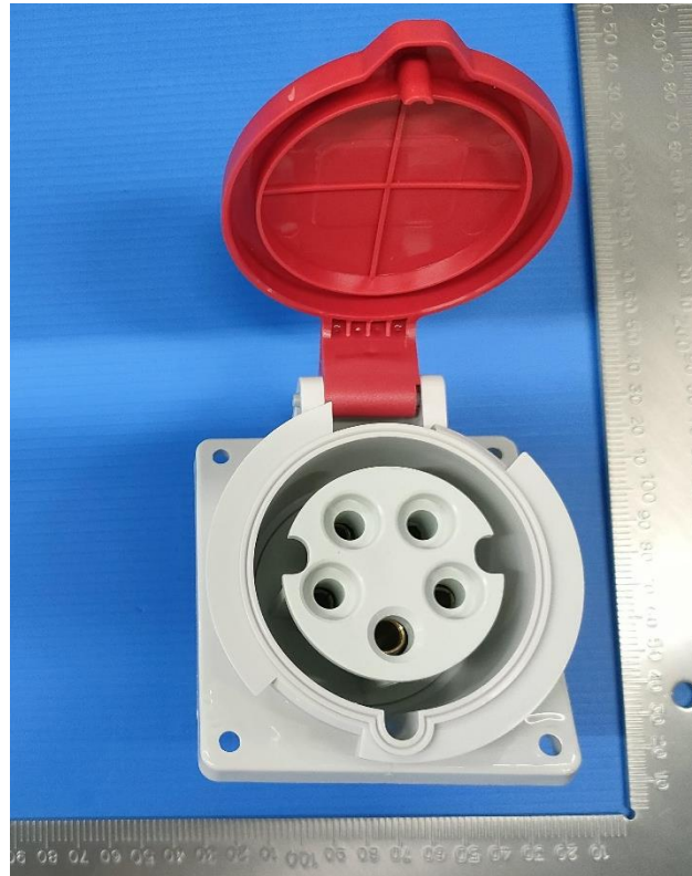
DEPU-425 32A-6h/415V ~ 3P+N+PE IP44
