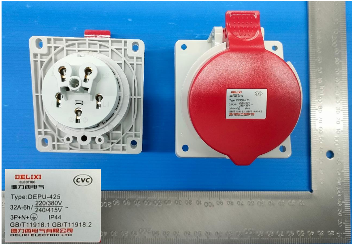
DEPU-425 32A-6h/415V ~ 3P+N+PE IP44
