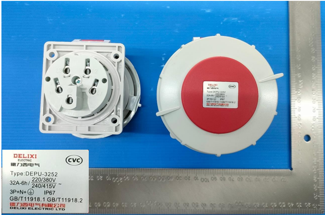
DEPU-3252 32A-6h/415V ~ 3P+N+PE IP67
