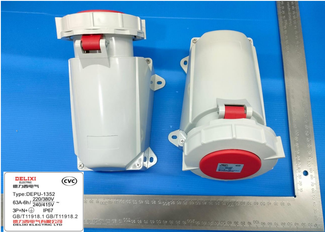
DEPU-1352 63A-6h/415V ~ 3P+N+PE IP67
