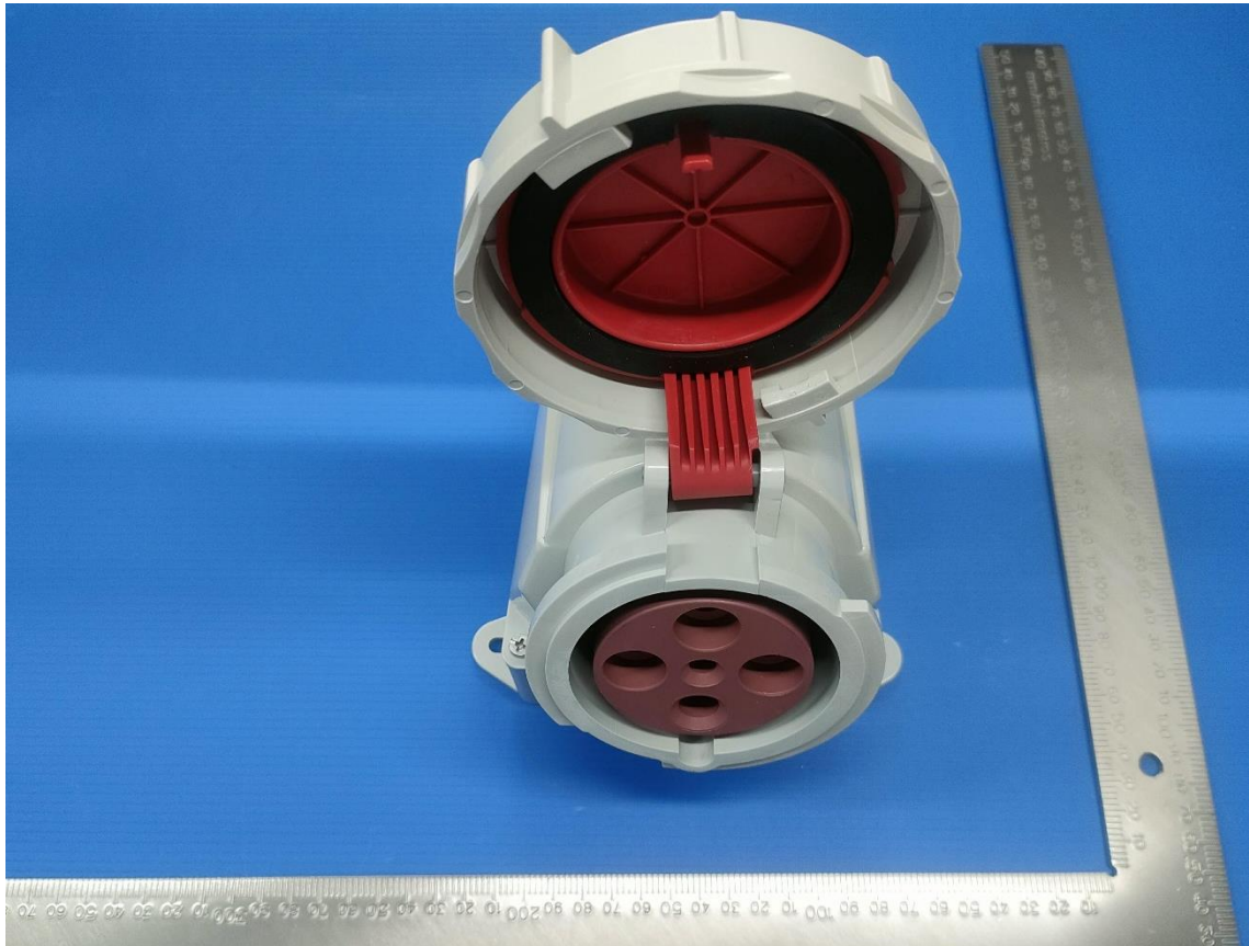
DEPU-1342 63A-6h/415V ~ 3P+PE IP67
