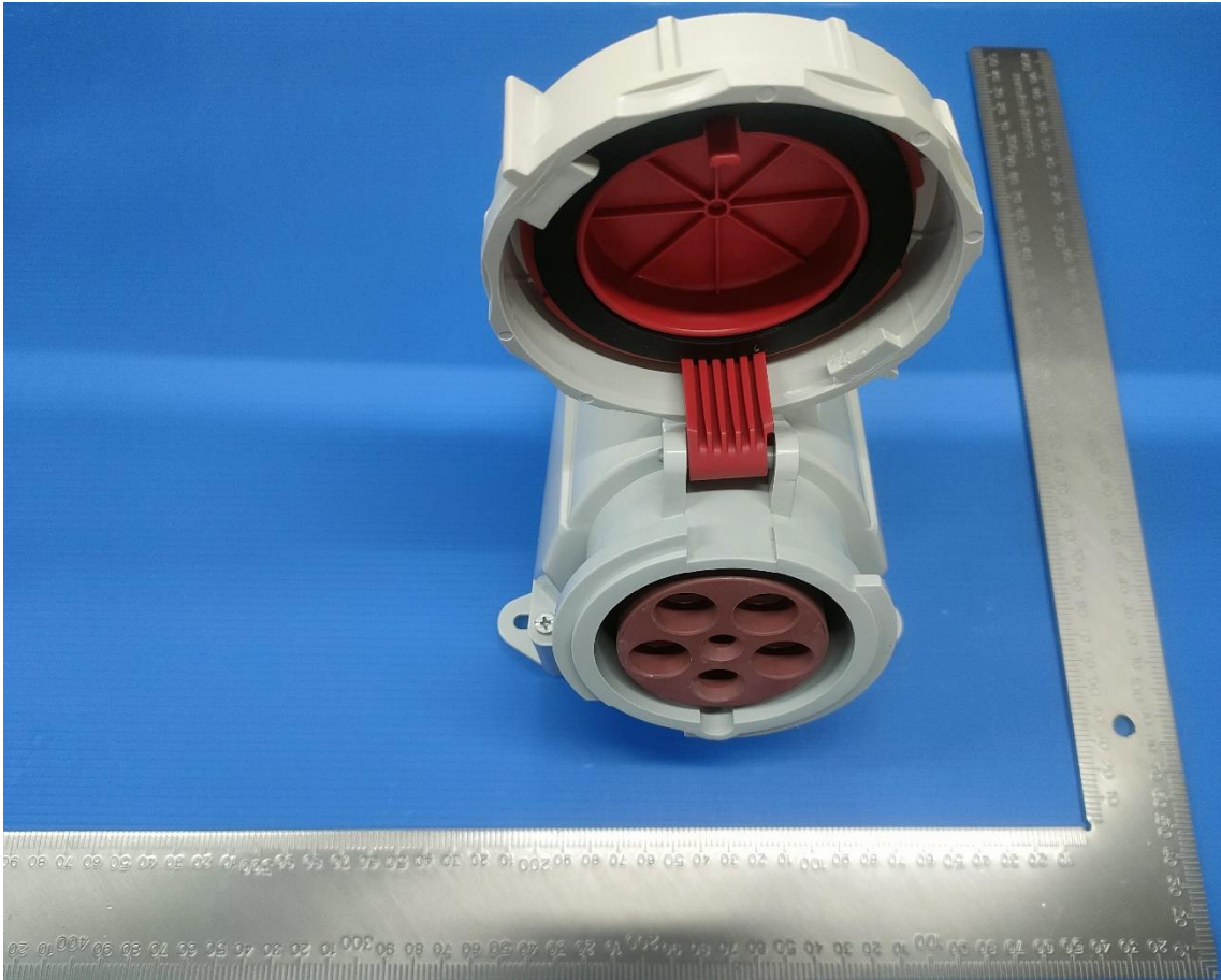
DEPU-1352 63A-6h/415V ~ 3P+N+PE IP67
