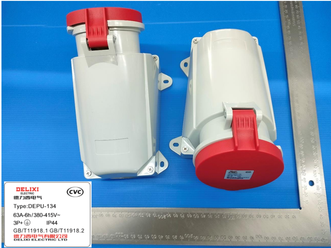
DEPU-134 63A-6h/415V ~ 3P+PE IP44
