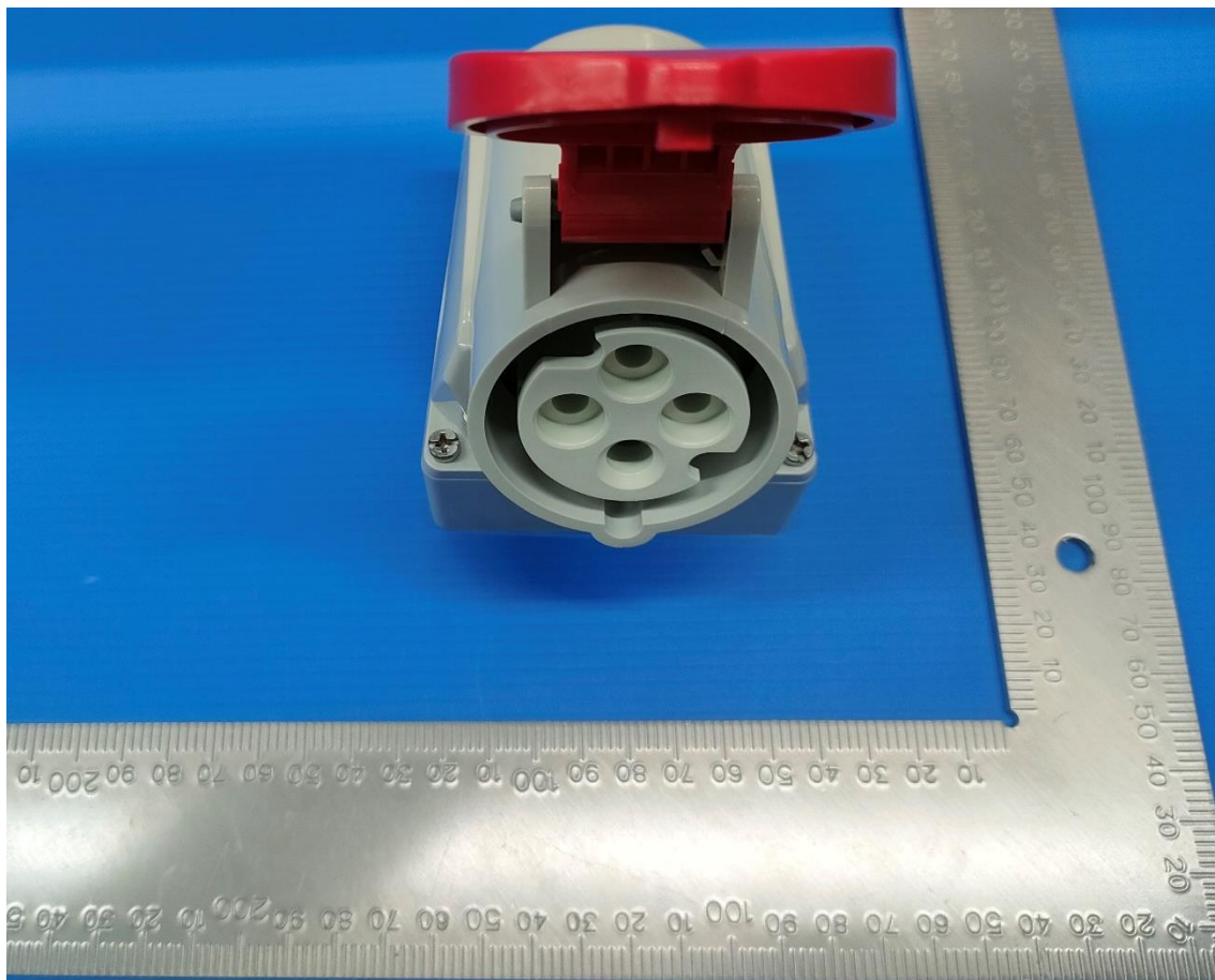
DEPU-114 16A-6h/415V ~ 3P+PE IP44
