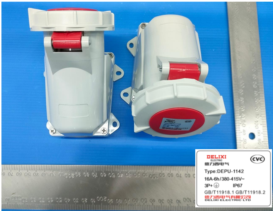
DEPU-1142 16A-6h/415V ~ 3P+PE IP67
