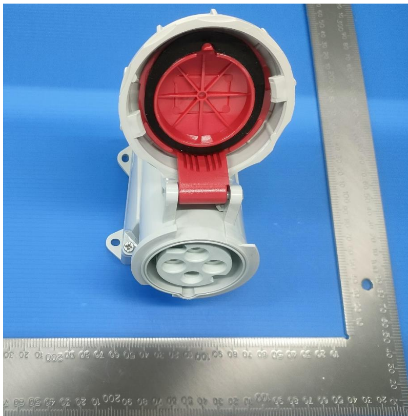
DEPU-1142 16A-6h/415V ~ 3P+PE IP67
