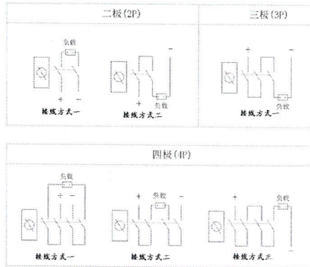
CEHS直流接线图
