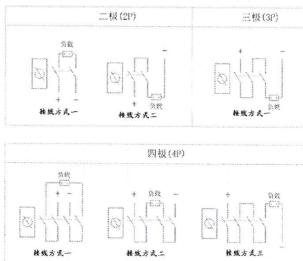
CDHS直流接线图
