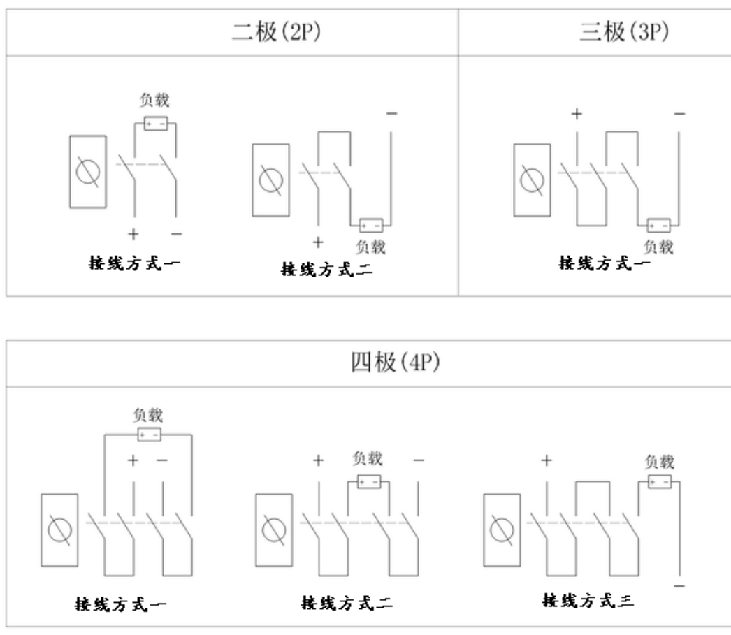
CDH8直流接线图
